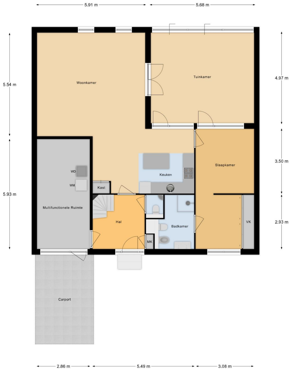
Begane Grond
